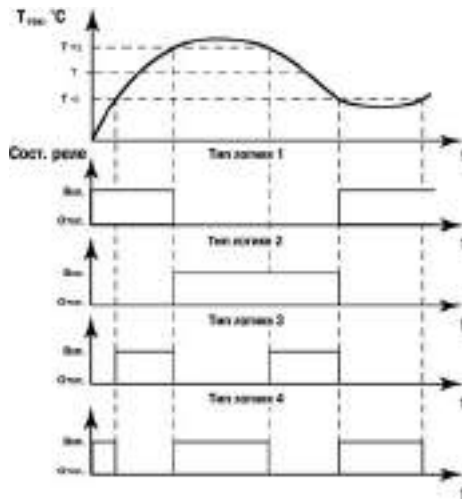
Рисунок 3.10 – Типы логики при работе ЛУ в режиме устройства сравнения
