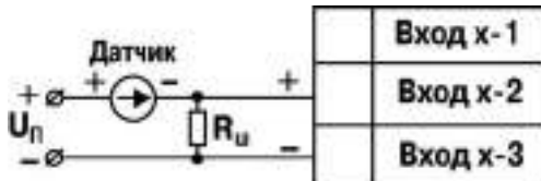
Рисунок Б.12 – Схема подключения активного датчика с токовым выходом 0...5 мА или 0(4)...20 мА R_{\text{ш}}=50,000 \pm 0,025 \text{ Ом}
